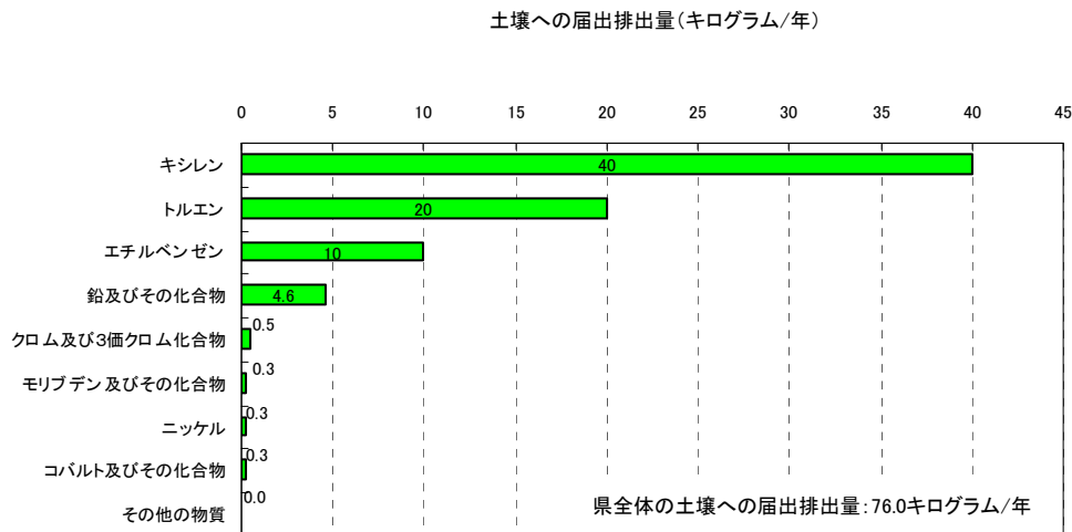
図 土壌への届出排出量
