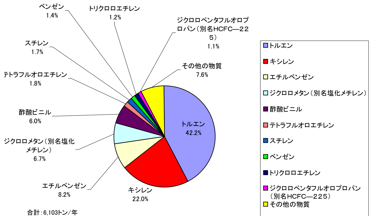
図 大気への届出排出量構成比
