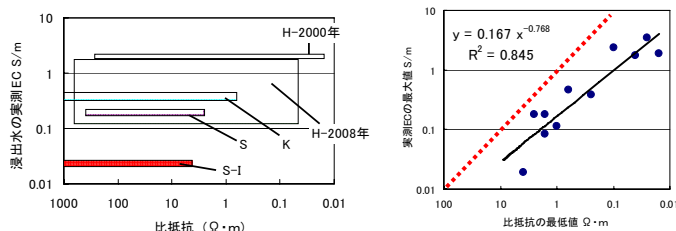
図3 浸出水 EC と比抵抗の比較2 図4 浸出水 EC と比抵抗の比較3
