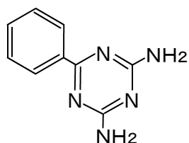
図1 構造式
