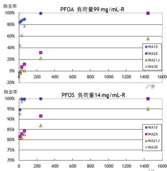
図1 バッチ処理による PFOA , PFOS の除去率
