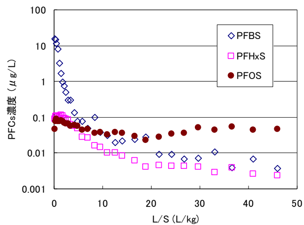
図 7-3 PFASs 濃度の変化(試料 A)
