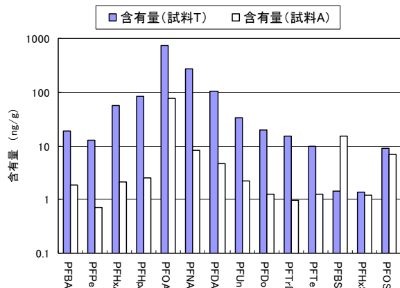
図5 試料の PFCs 含有量 (ng/g)
