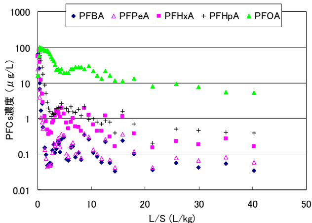
図 6-1 PFCAs 濃度の変化 1 (試料 T)
