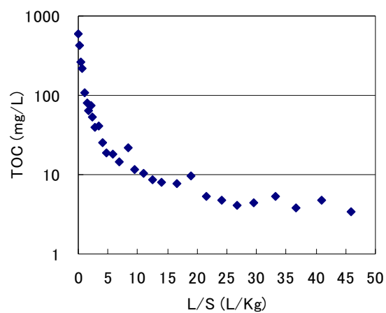
図 7-5 TOC 濃度の変化(試料 A)
