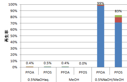
図17 溶液毎の樹脂の再生率
