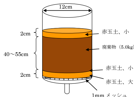
図1 廃棄物カラムの充填方法
