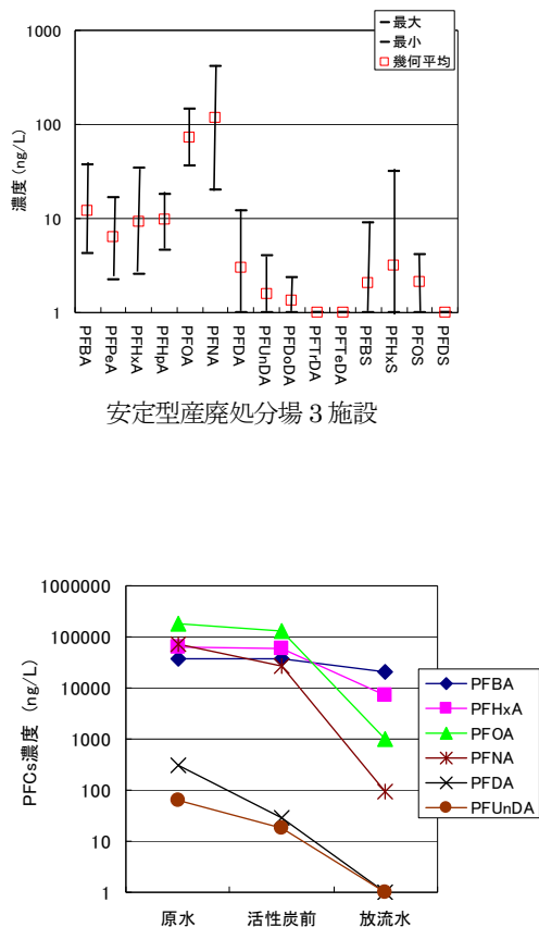
図5 水処理による濃度変化
