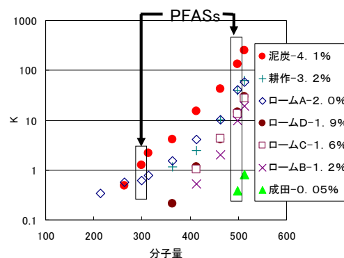
図 1 2 PFCs の分子量と分配定数の比較
