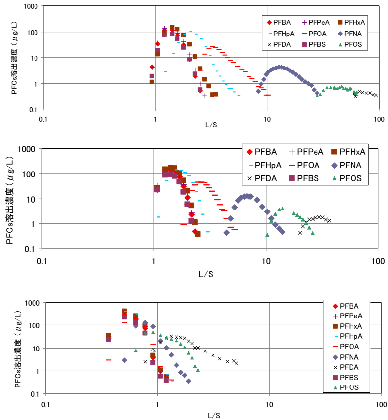
図9 PFCs 溶出濃度 (上からローム A, ローム B, 成田)
