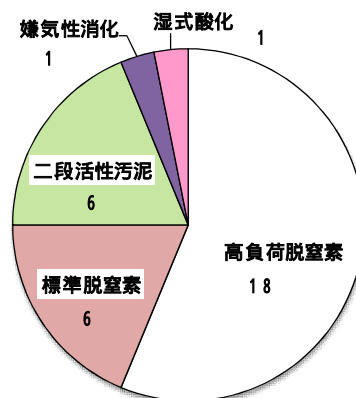
図1 千葉県の上尿処理施設の主処理の内訳 (2012年度届出 32施設)
