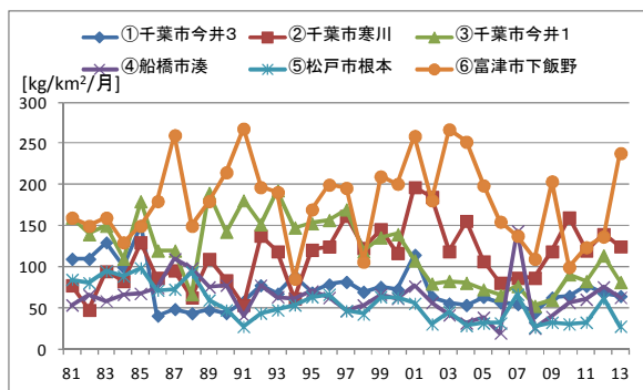
図5 Al 降下量の経年推移
