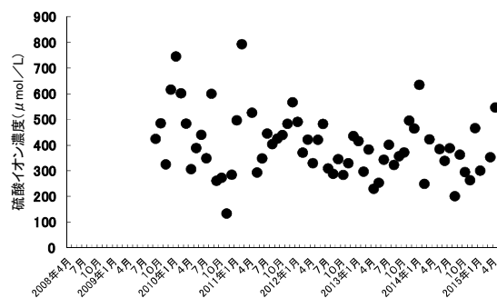
図4 キンダン川渓流水 \text{SO}_4^{2-} 濃度 ( \mu\text{mol L}^{-1} )
