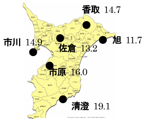
図1 降水中 \text{nss-SO}_4^{2-} 濃度分布 ( \mu\text{mol L}^{-1} ) (2008~2012年度平均)
