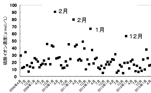
図3 清澄降水中 \text{nss-SO}_4^{2-} 濃度 ( \mu\text{mol L}^{-1} )
