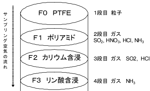
図2 フィルターパック法
