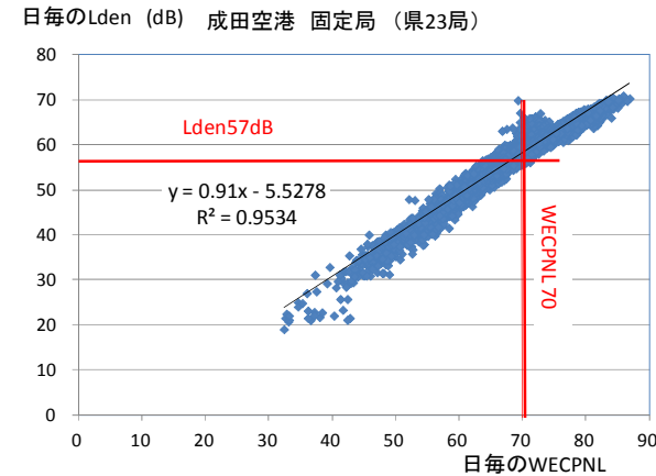
図1 WECPNL と Lden の関係（成田空港・2013）
