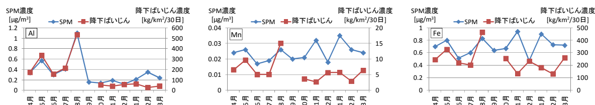
図5 富津下飯野における降下ばいじん及びSPM中のAl及びFe濃度の推移（2014年度）
