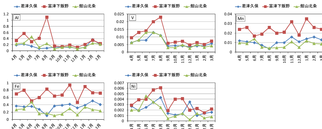
図4 浮遊粒子状物質調査（2014年度）におけるAl、Fe月平均濃度推移(µg/m³)
