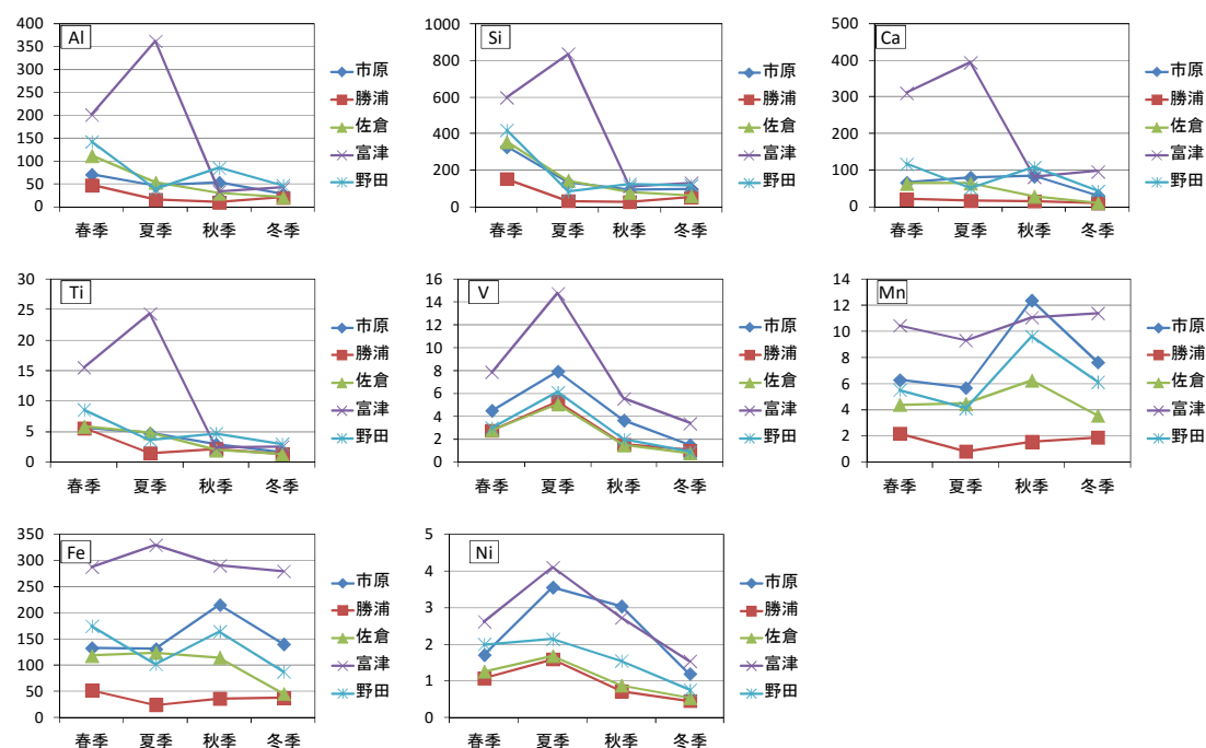
図3 富津下飯野において高濃度となった指標元素の濃度推移(ng/m 3 )
