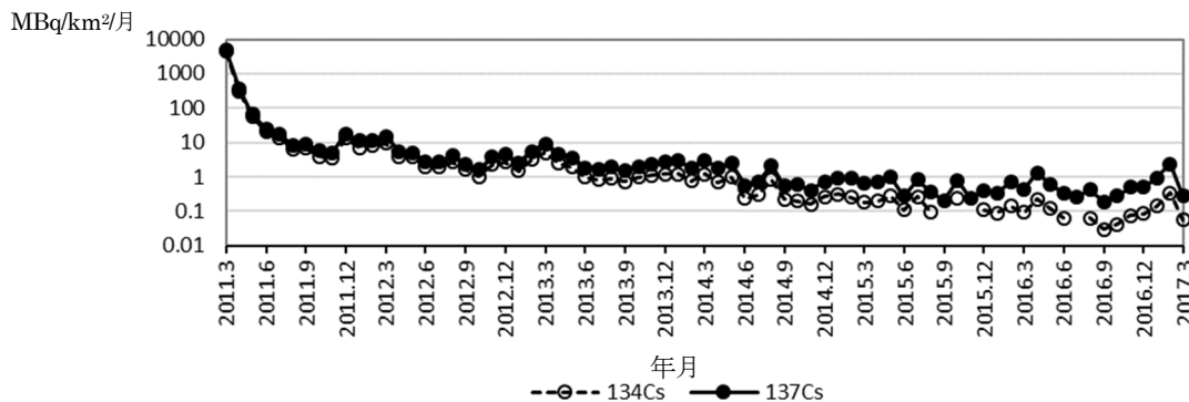
図1 月間降下物中の ^{134}\text{Cs} 及び ^{137}\text{Cs} 量
