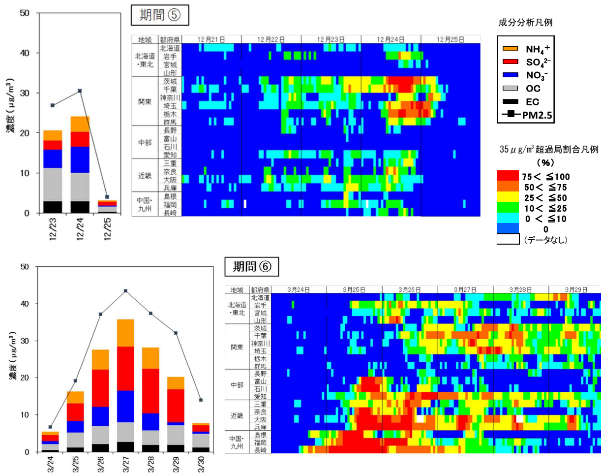
図1 主要5成分の濃度推移及び全国のPM2.5の高濃度状況
