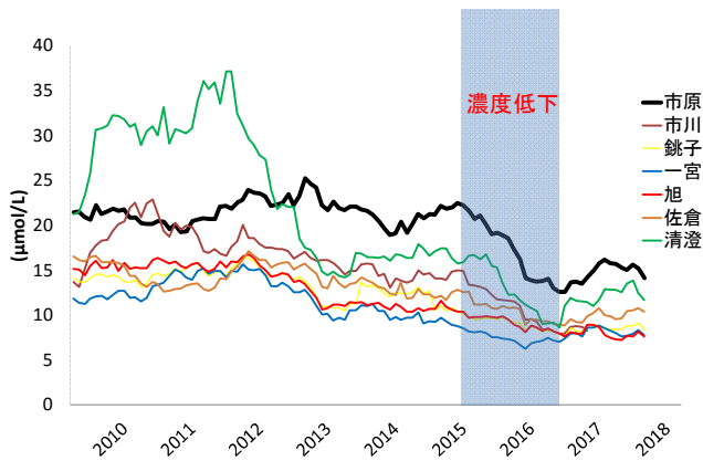
図1 降水中 \text{nss-SO}_4^{2-} 濃度推移
