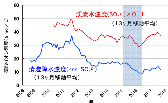
図4 渓流水 \text{SO}_4^{2-} 濃度と降水中 \text{nss-SO}_4^{2-} 濃度
