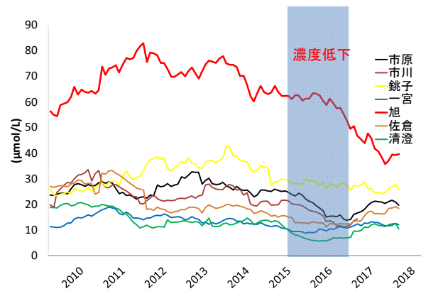
図2 降水中 \text{NH}_4^+ 濃度推移
