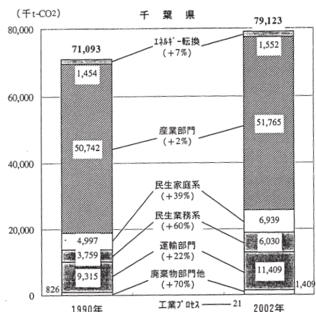
図2-3-2 千葉県内の部門別二酸化炭素排出量の推移
