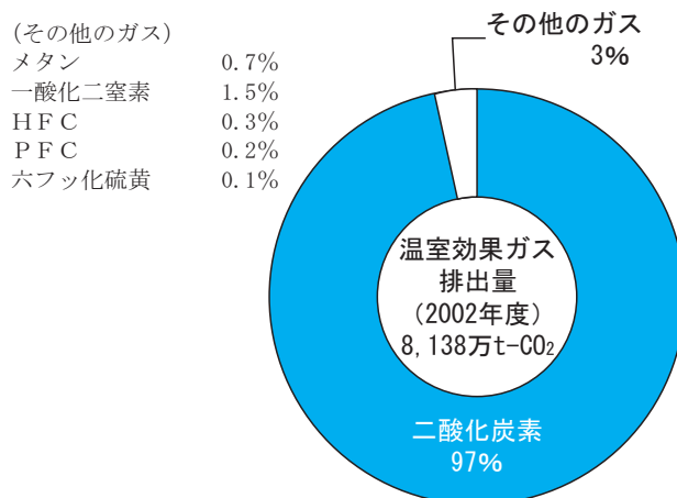
図2-3-1 千葉県内の温室効果ガスの排出割合（2002年度）
